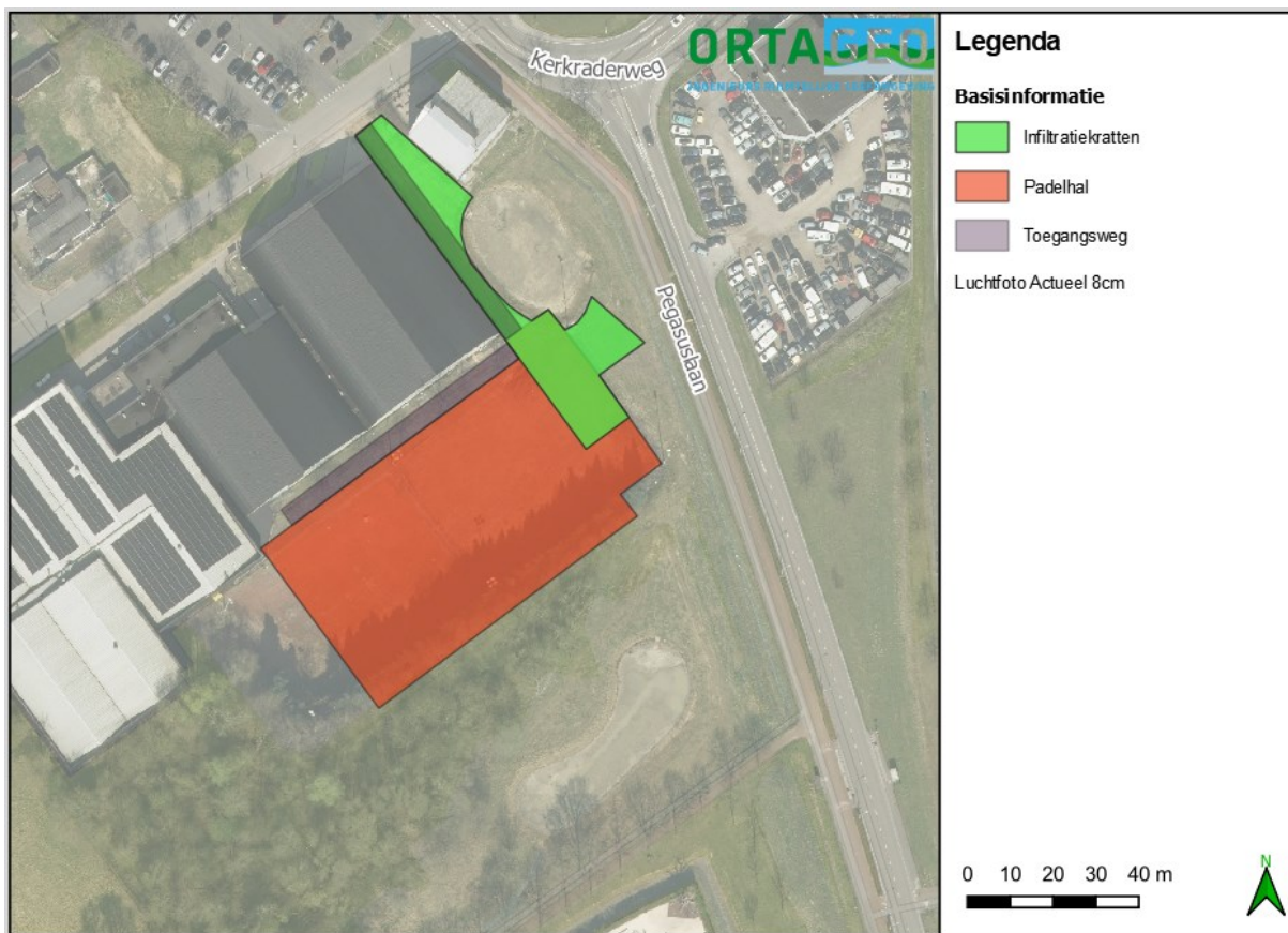
Afbeelding 2: Toekomstige situatie: infiltratiekratten, padelhal en wegen (bronnen 3A en 4A)
