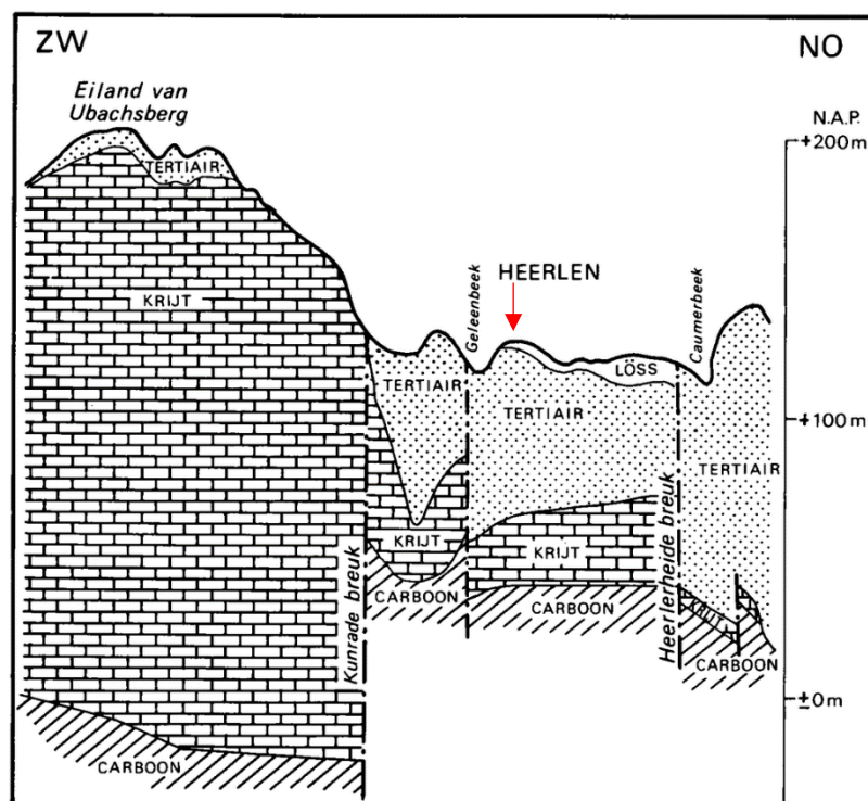
Figuur 3. Schematische doorsnede van het Bekken van Heerlen met de ligging van het plangebied bij benadering aangegeven door een rode pijl (Bosch, 1987).
