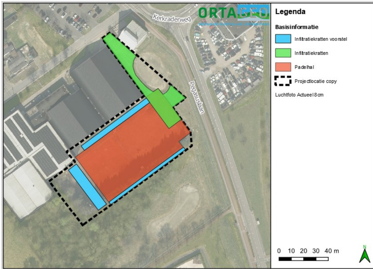
Afbeelding 3: Voorstel extra infiltratie kratten
