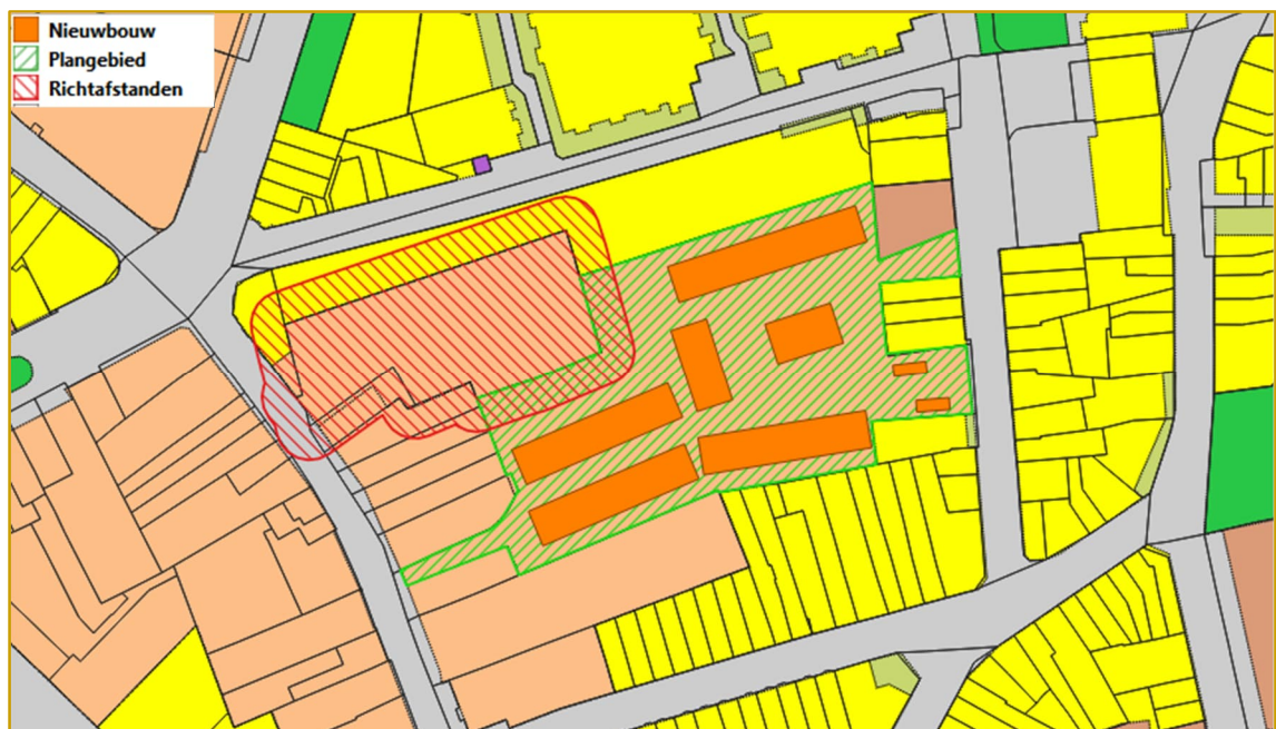
Afbeelding 4 Richtafstanden omliggende percelen
