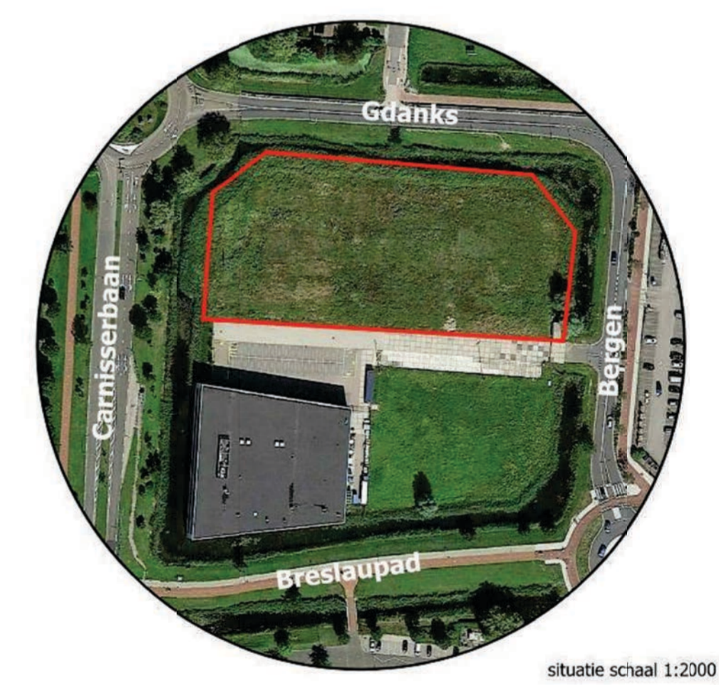
situatie schaal 1:2000
