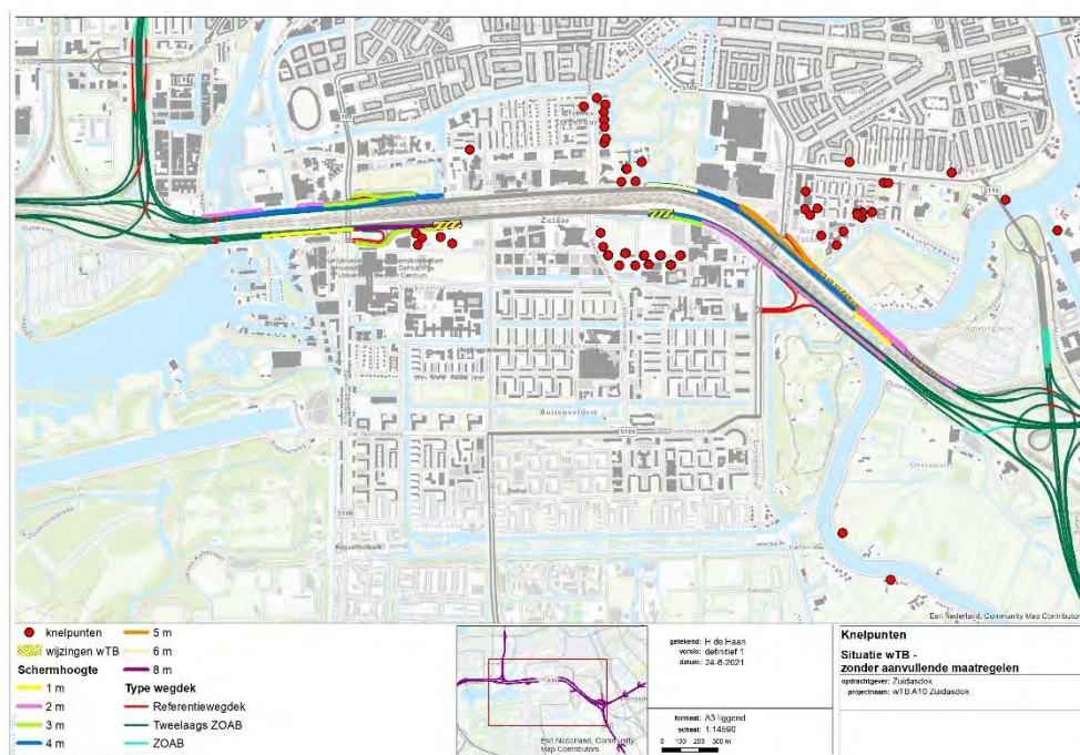
Figuur 42. Ligging van geluidgevoelige objecten met een toename van de geluidbelasting
