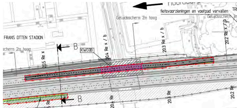
Figuur 4 Wijziging 12 met rechts invoegende rijstrook
