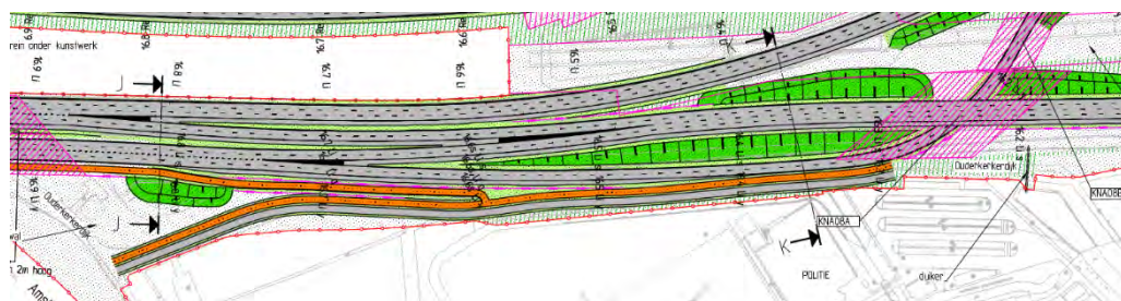
Figuur 12 TB kaart met losliggend fietspad
