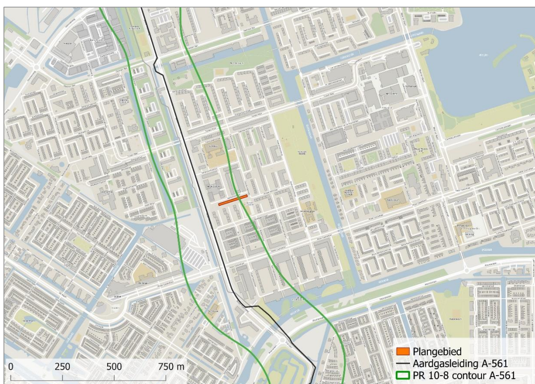
Figuur 2. PR-contour aardgasleiding A-561
