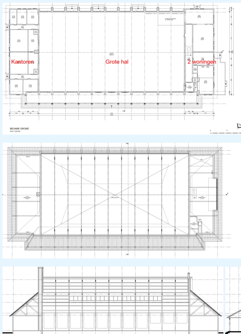
figuur 3: plattegronden en doorsneden
