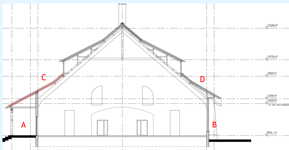
figuur 4: meetposities uitwendige schil
