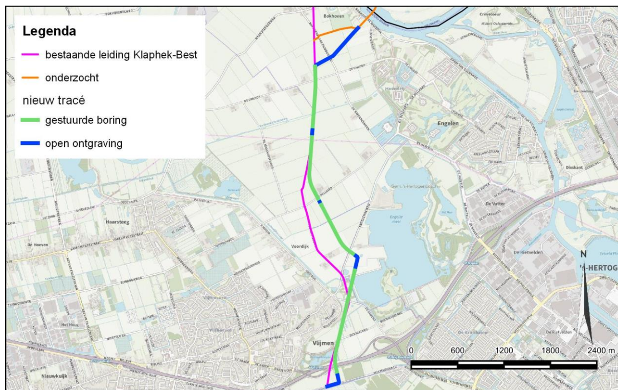
Figuur 2: Het huidige en nieuwe tracé van de brandstofleiding.
