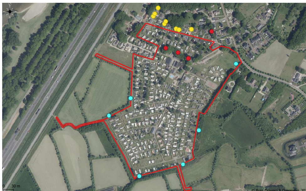
Figuur 4. Locaties tijdelijke voorzieningen voor gewone dwergvleermuis: 8 vleermuiskasten type VK WS 02 of VK WS 11 van Vivara Pro aan gevels (gele stippen), 4 vleermuiskasten type VK WS 04 van Vivara Pro aan bomen (rode stippen) en 12 vleermuiskasten type 1FF van Schwegler aan palen (blauwe stippen).
