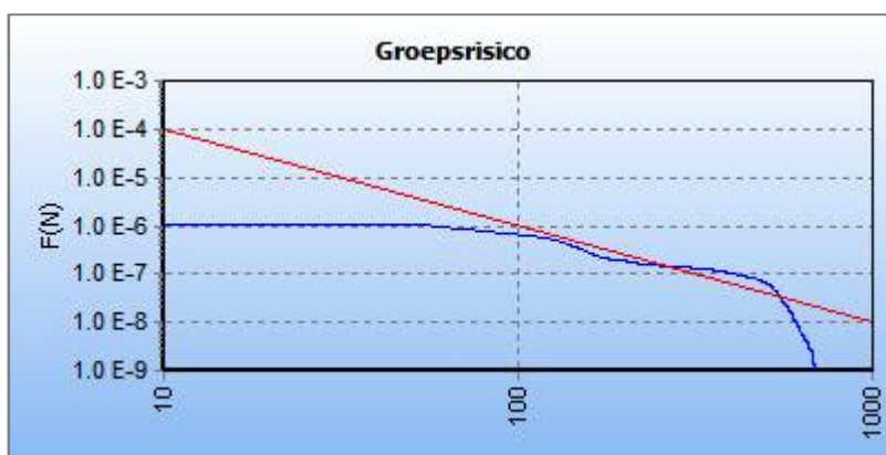
Figuur 7. 2. Leiding A-510, huidige en toekomstig situatie
