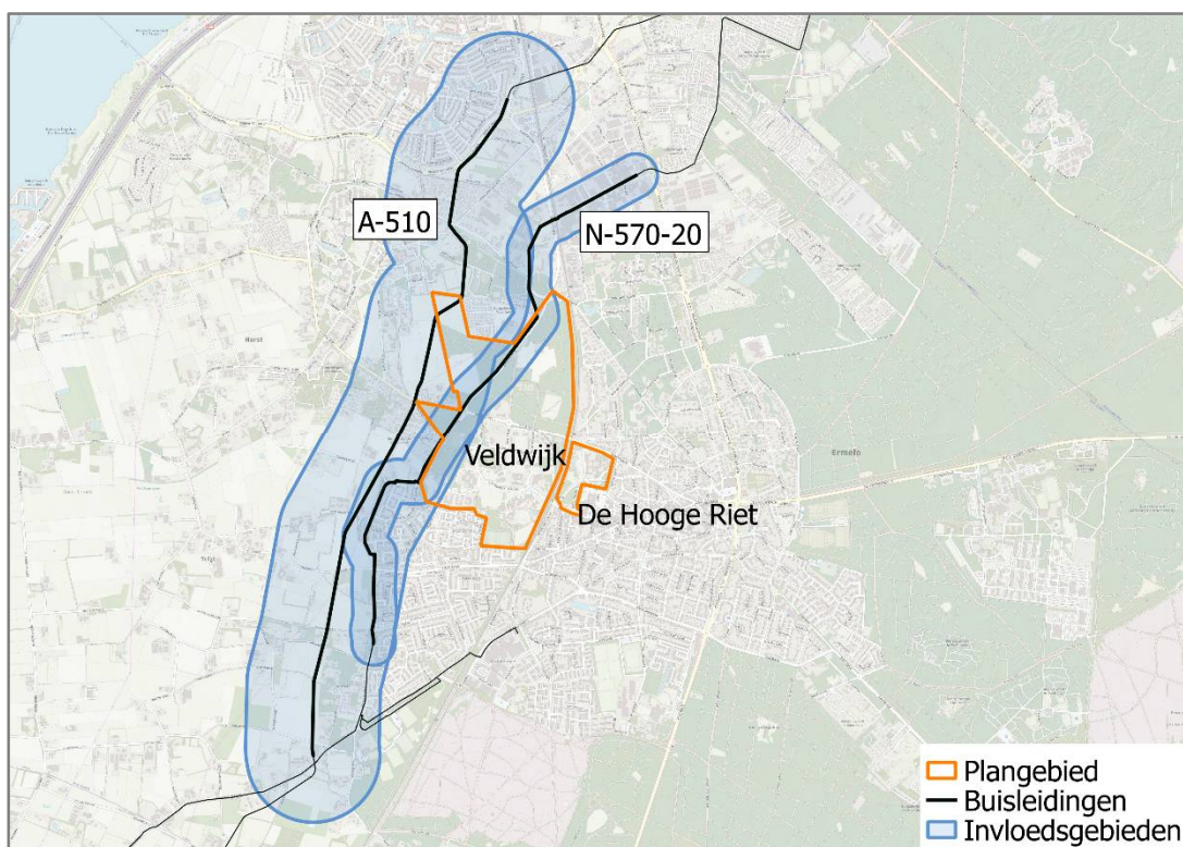
Figuur 3. Aardgasleidingen en invloedsgebieden
