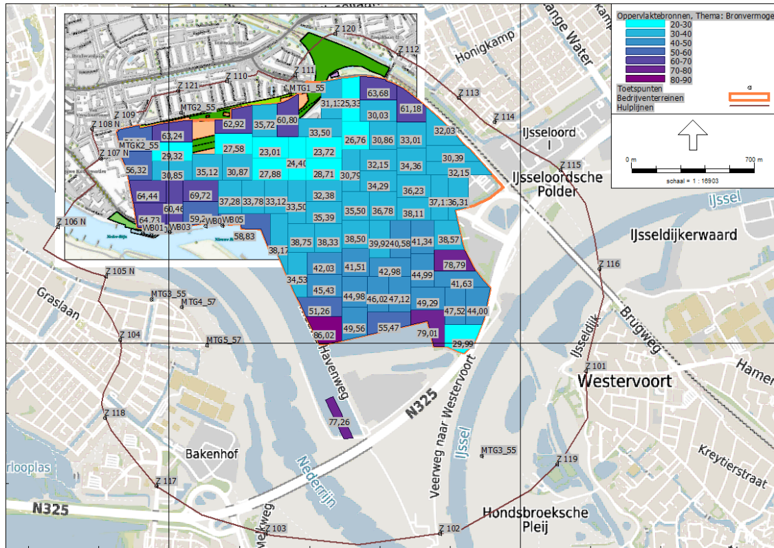
figuur 8: maximale invulling hele industrieterrein. Bronvermogen per m2 van lichtblauw (20 dB(A)/m2) naar paars (90 dB(A)/m2). De oranje lijn is de industriegrens en de bruine lijn is de 50 dB(A) geluidcontour.
