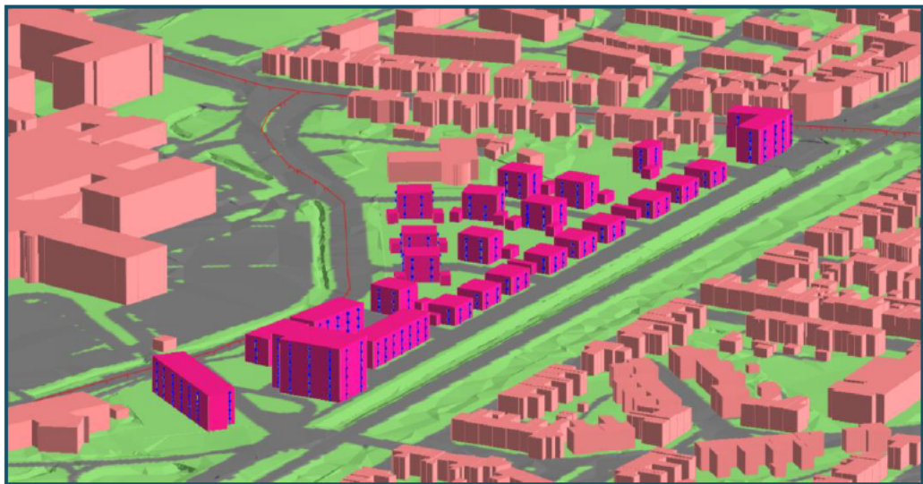
Figuur 6 Impressie rekenmodel wegverkeerslawaaai
