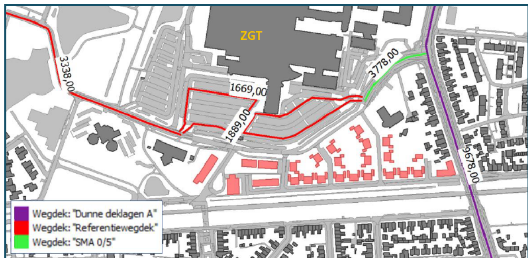
Figuur 5 Etmaalintensiteiten en verhardingsgegevens wegen 2040
