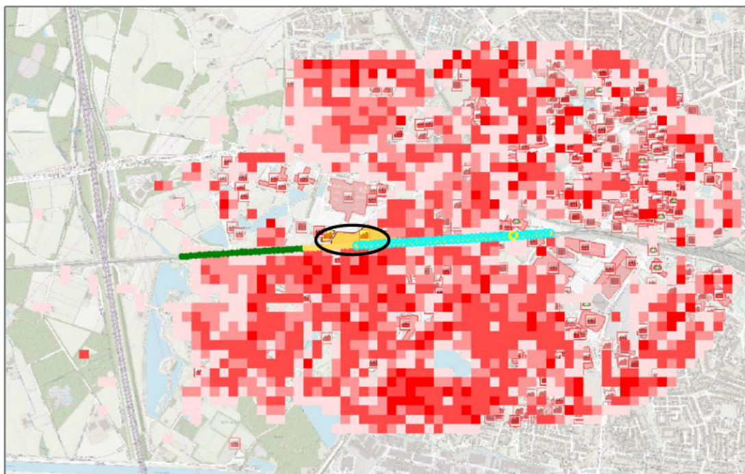
Figuur 4. Geografische weergave GR spoorlijn Delden - Hengelo, toekomstige situatie
