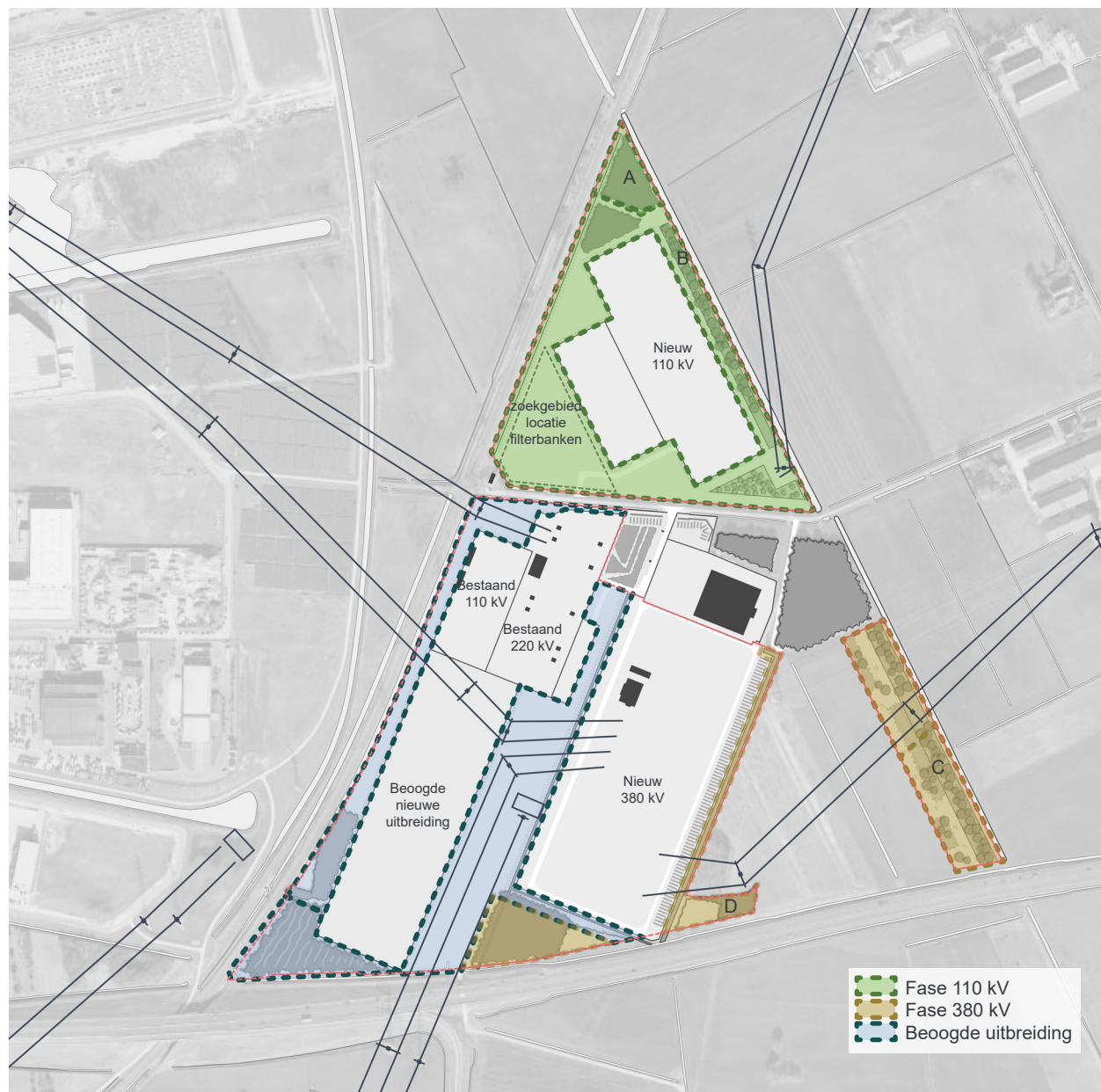
Afbeelding 5.21 fasering
