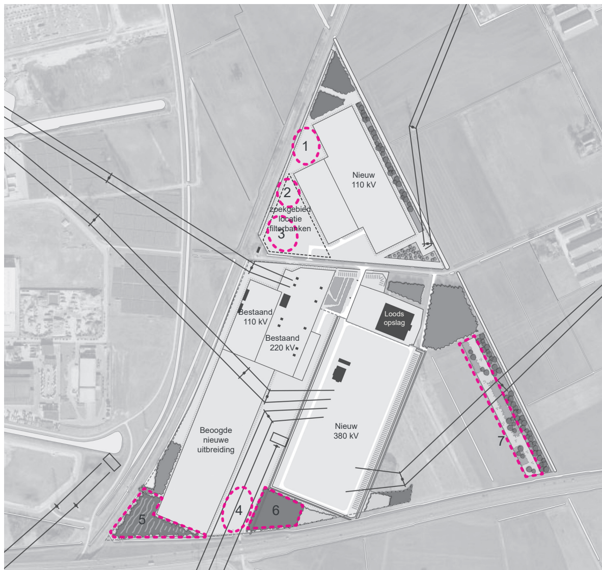
Afbeelding 5.19 opgave water
