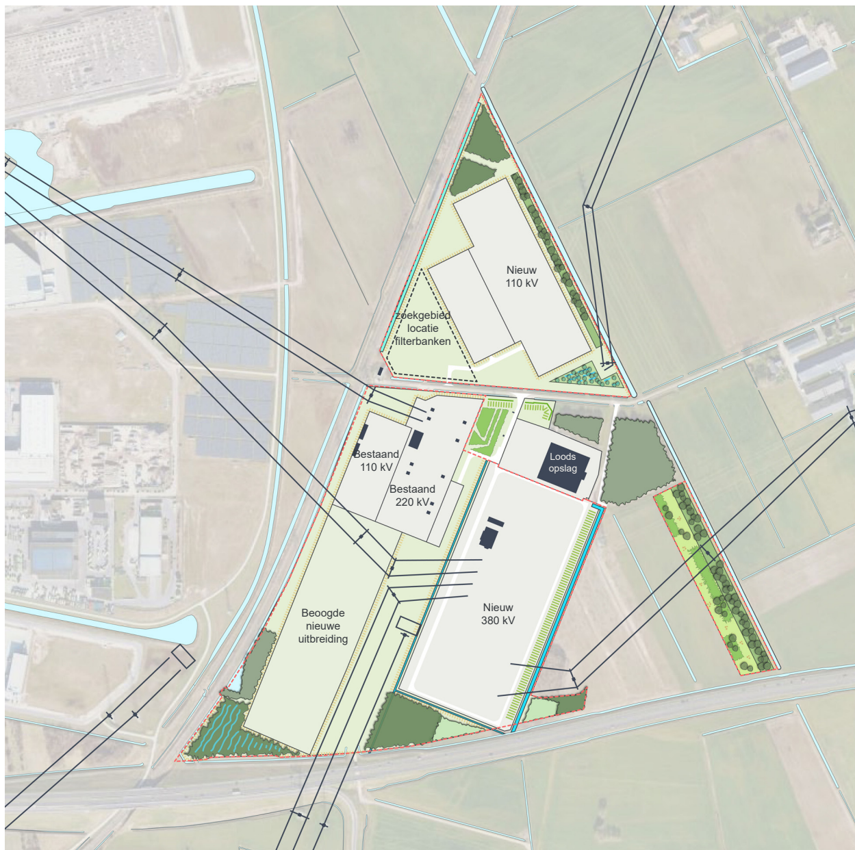
Afbeelding 5.1 landschappelijk inpassingsplan
