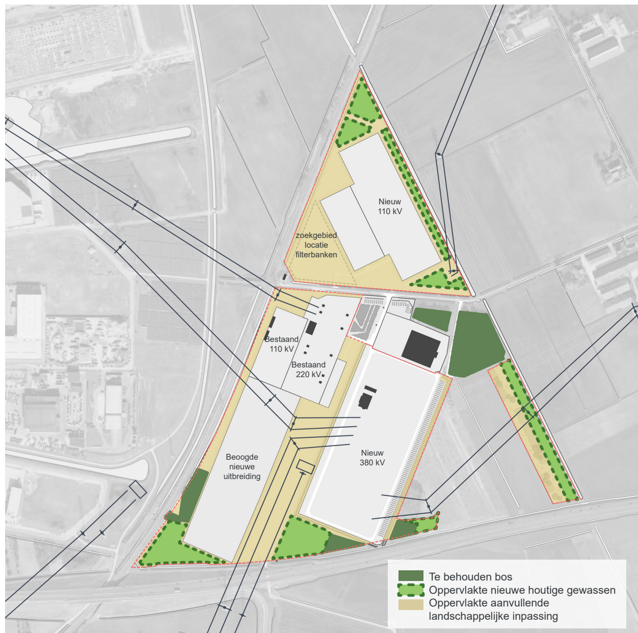
Afbeelding 5.18 kwantitatieve opgave
