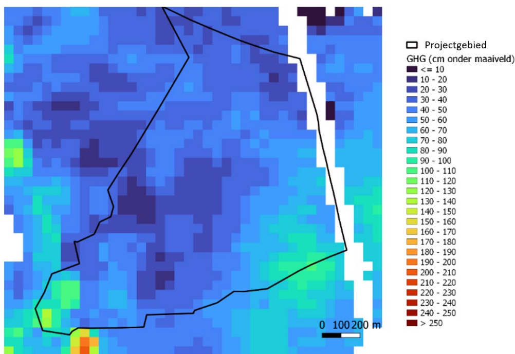
Figuur 2-5. De gemiddeld hoogste grondwaterstand (GHG) in het projectgebied (zwart omlijnd) op basis van simulaties met een landelijk grondwatermodel gepresenteerd op het Dinoloket .
