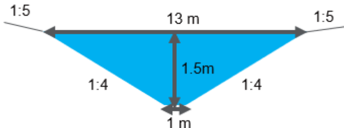
Figuur 32 Schematische weergave huidige Kievitstocht.
